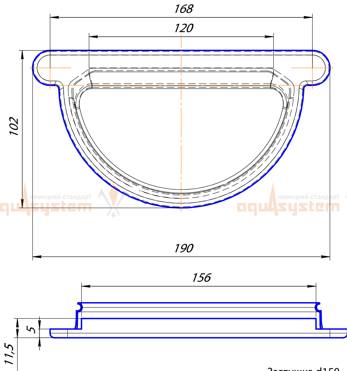
Заглушка d150
