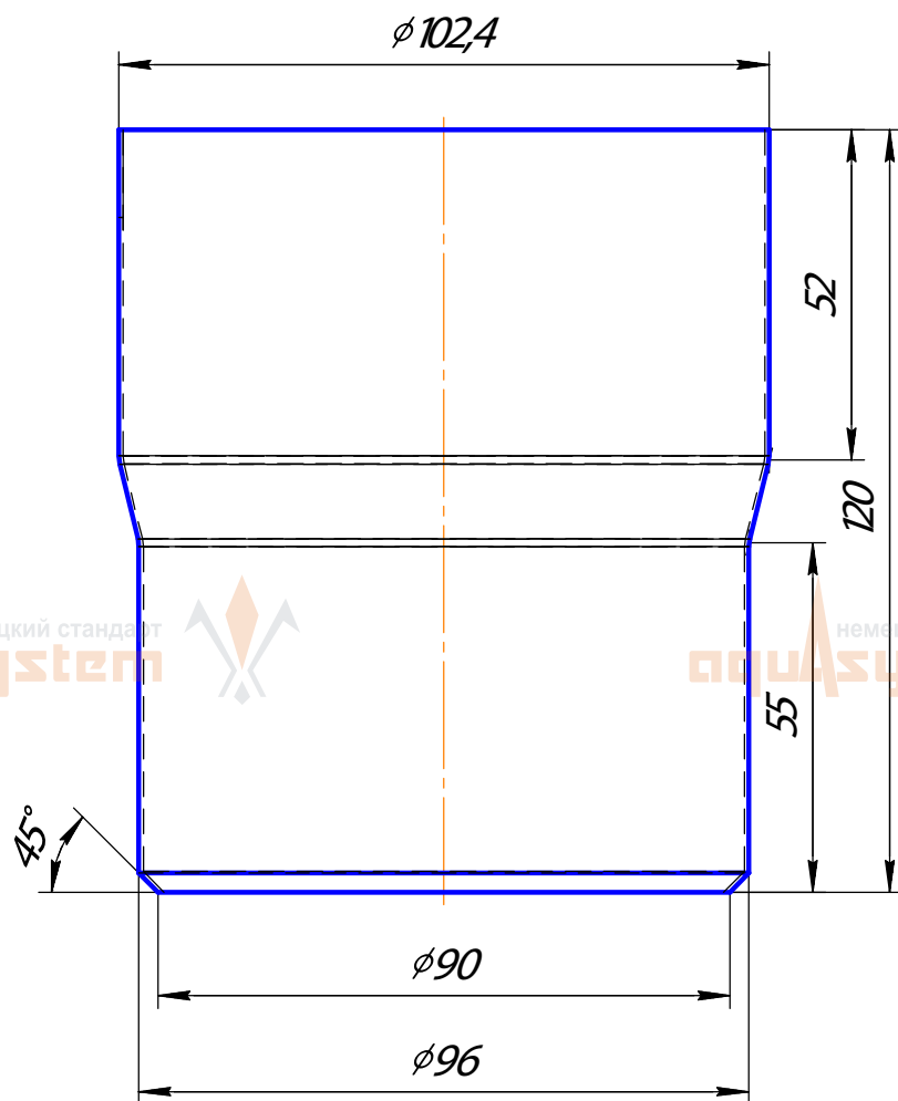
Соединитель трубы d100
