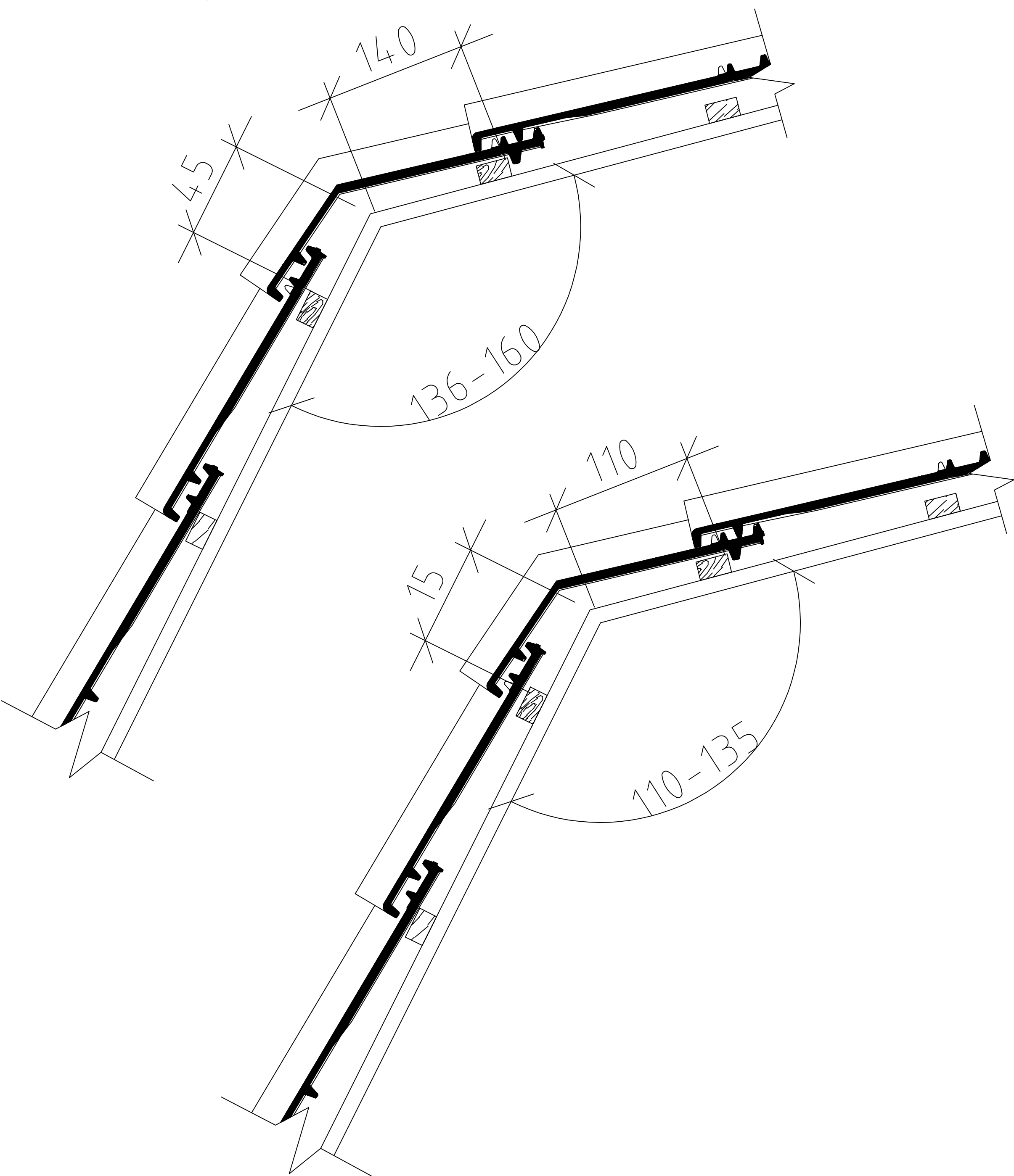
Выпуклая мансардная черепица
